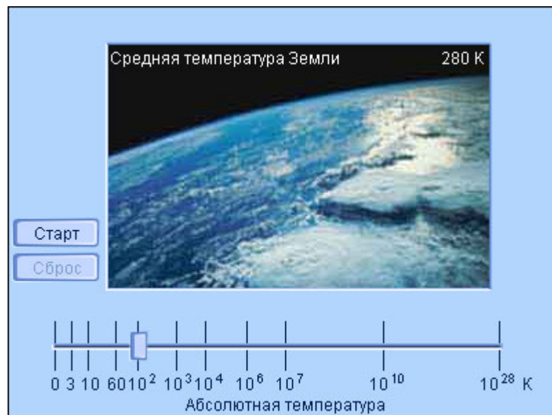
Модель 2.5. Абсолютная температура
