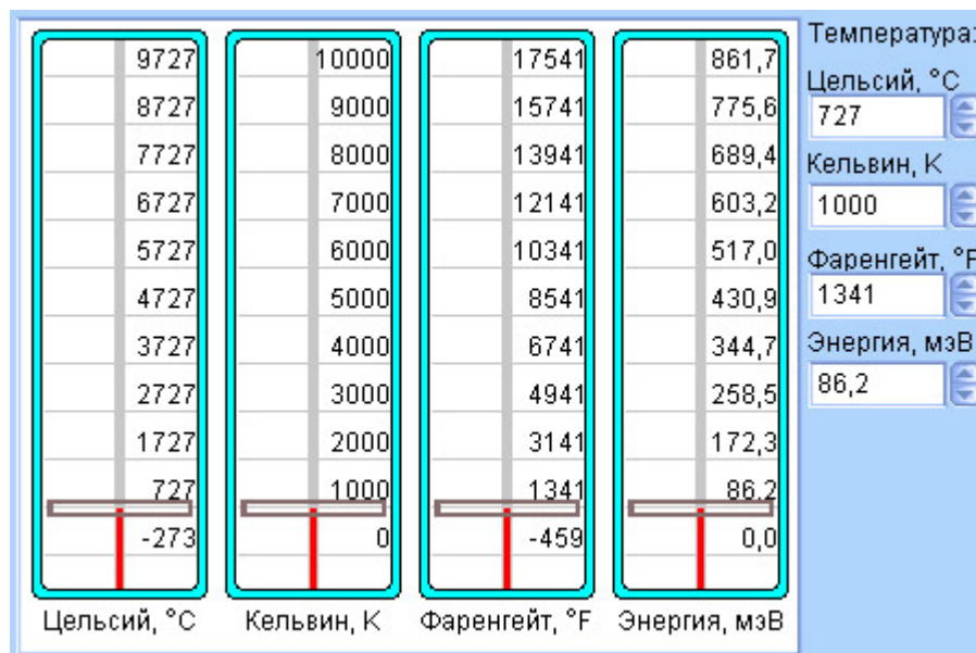
Модель 2.6. Температурные шкалы
